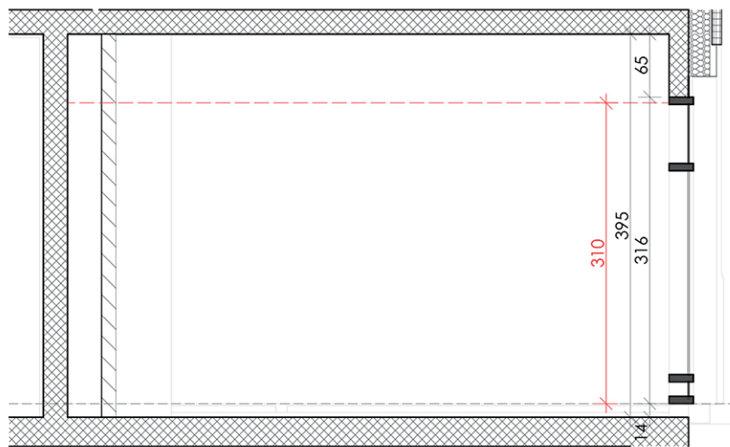
COUPE A-A
