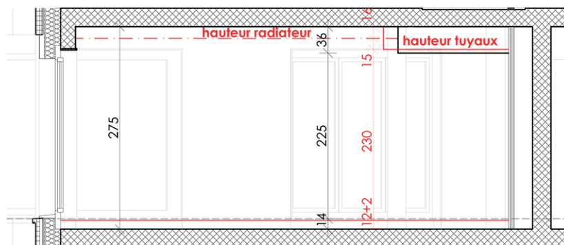
COUPE B-B
