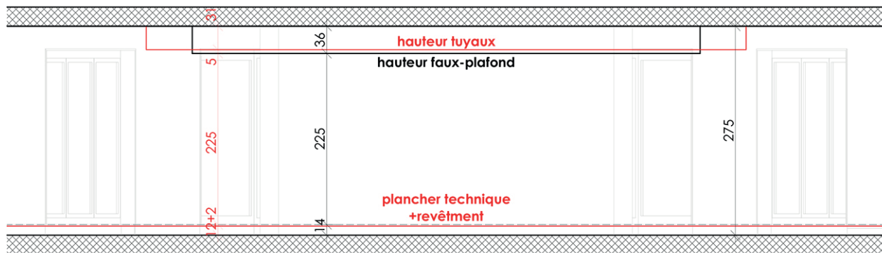
COUPE A-A
