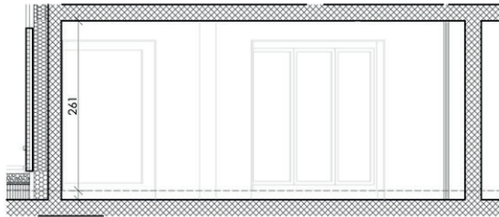
COUPE A-A
